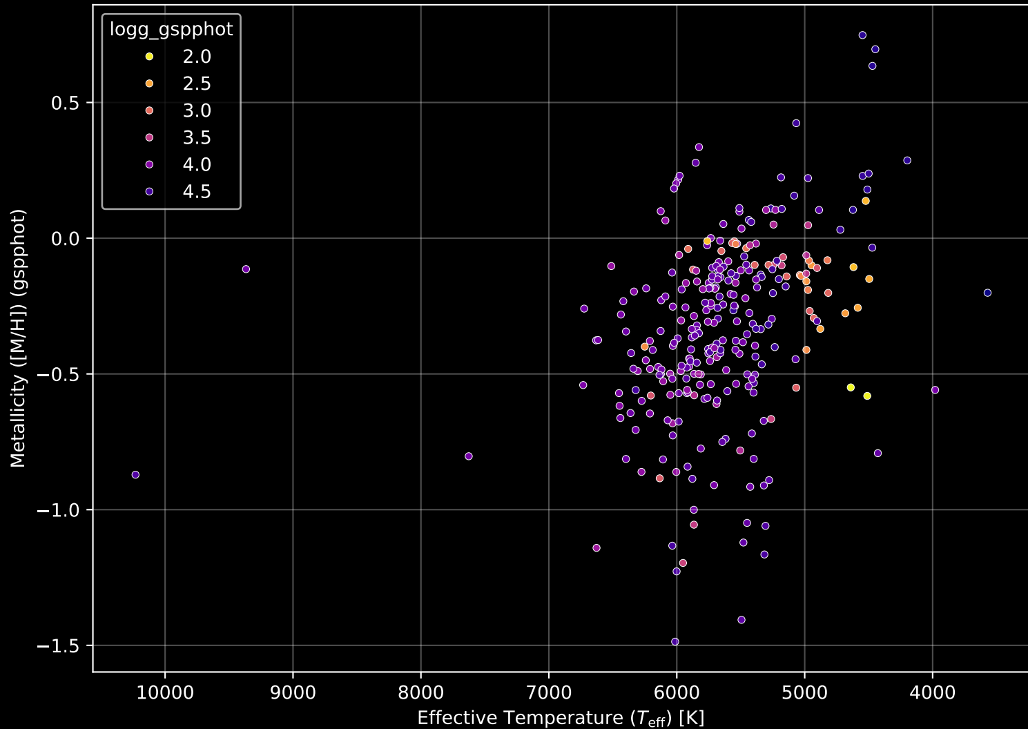
GALAH DR4 Field: [728] Stellar Population Parameters (n= 292)
