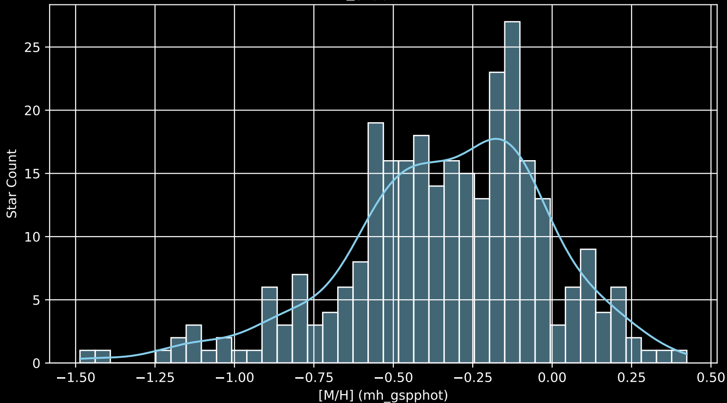
GALAH DR4 Field: [728] [M/H] (mh_gspphot) (n= 289)
