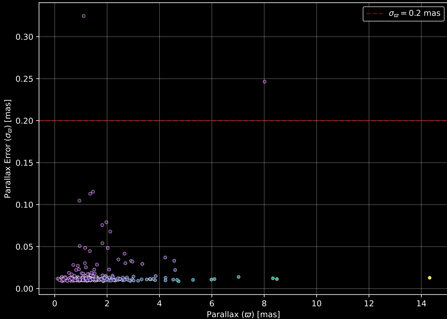
GALAH DR4 Field: [728] Parallax Quality (n= 292)
